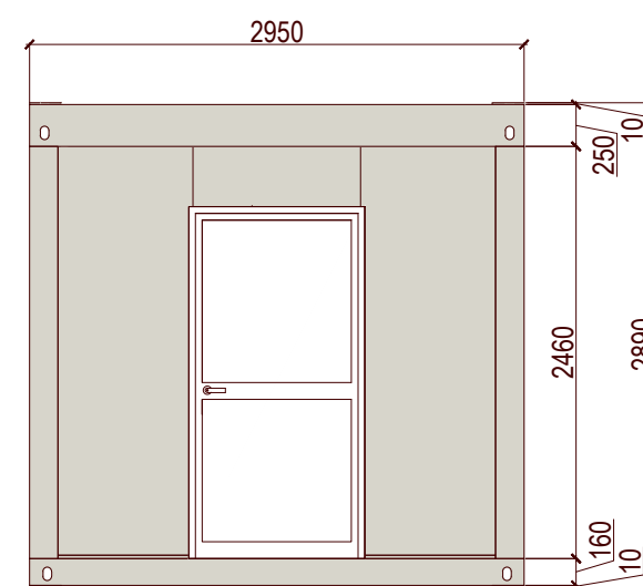
ÉLÉVATION "D"
