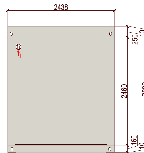
ÉLÉVATION "B"
