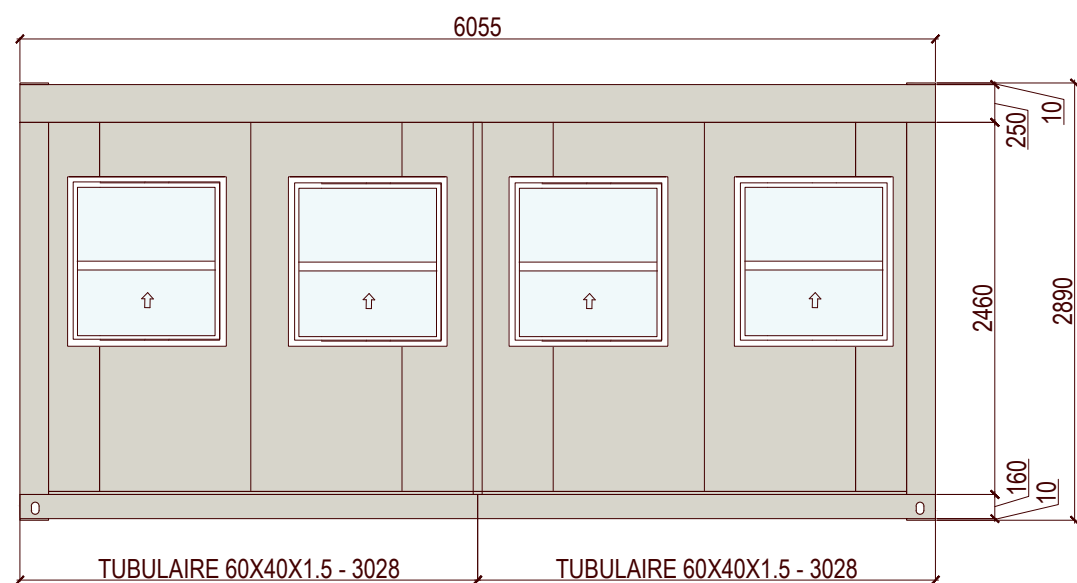
ÉLÉVATION "A"
