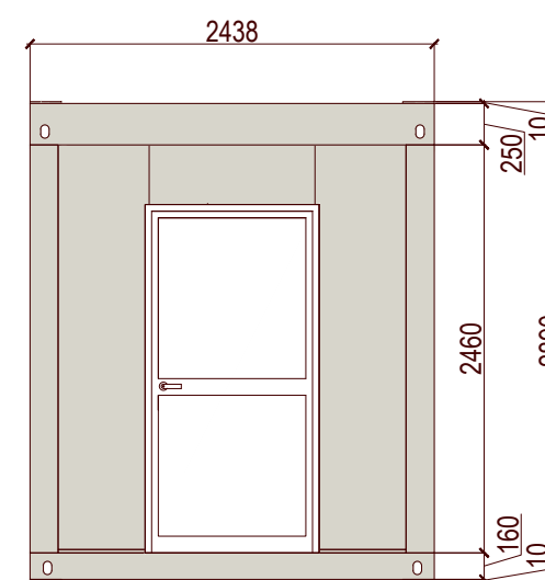
ÉLÉVATION "D"
