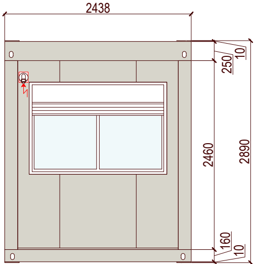
ÉLÉVATION "B"
