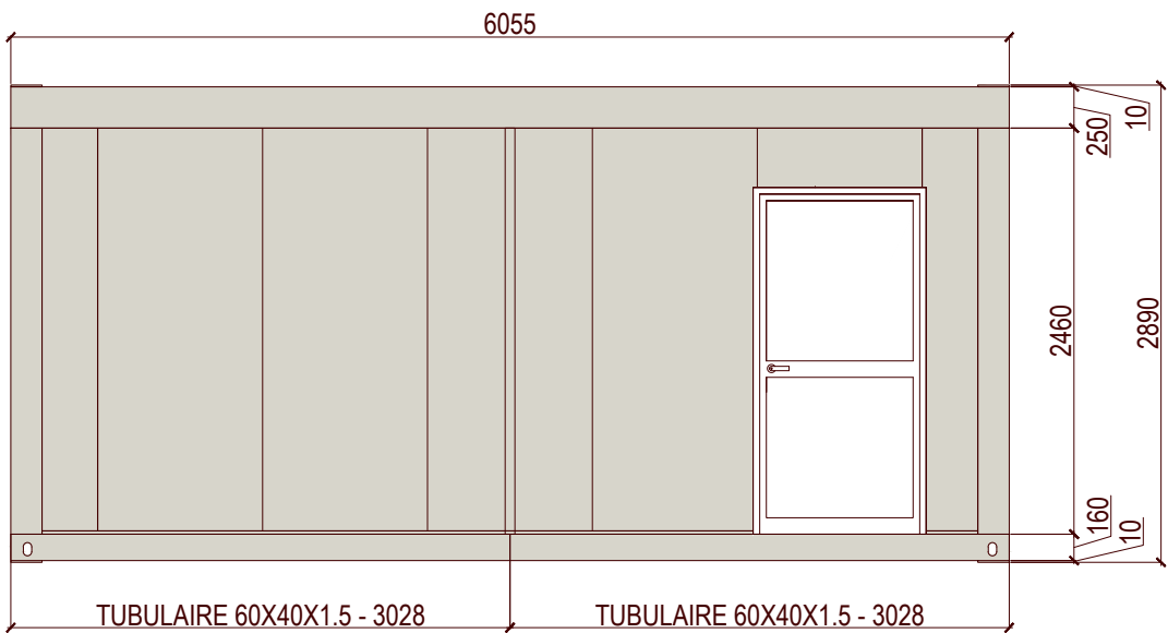
ÉLÉVATION "A"
