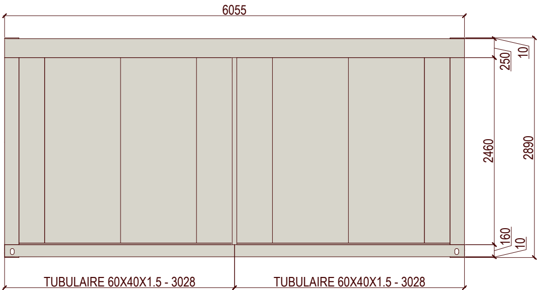
ÉLÉVATION "C"
