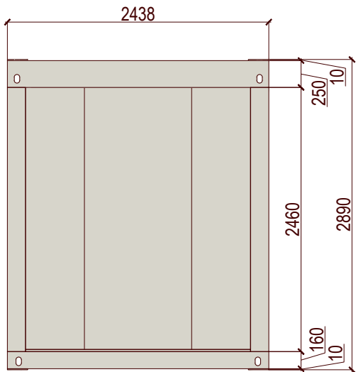
ÉLÉVATION "D"
