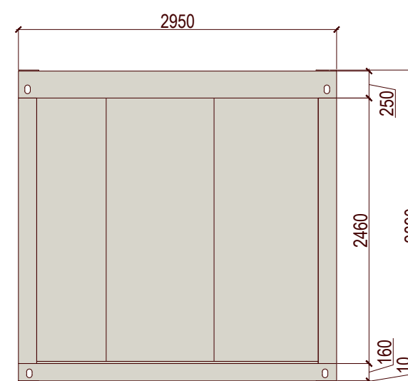
ÉLÉVATION "B"
