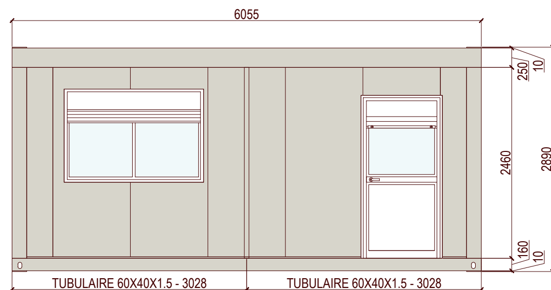
ÉLÉVATION "A"
