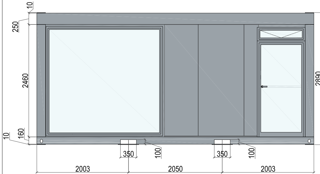
ÉLÉVATION "A"
