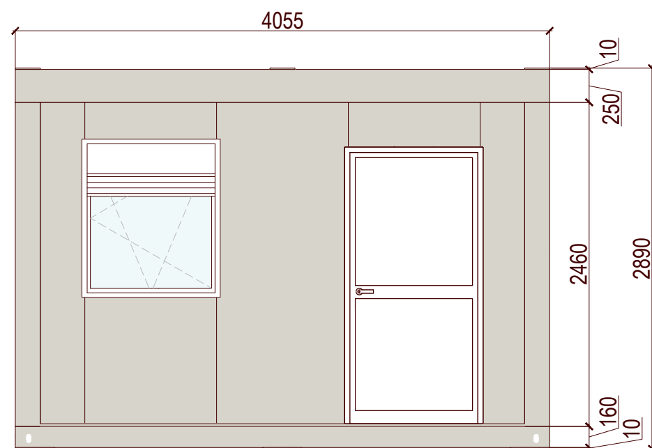
ÉLÉVATION "A"
