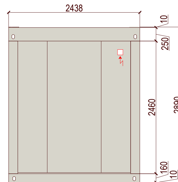
ÉLÉVATION "D"
